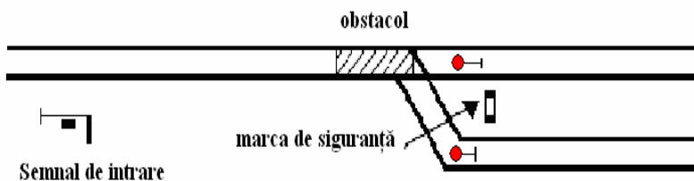
Fig. 5. Acoperirea unui obstacol sau a locului de executare a lucrării, dacă acesta se află pe schimbătorul de cale de intrare.
