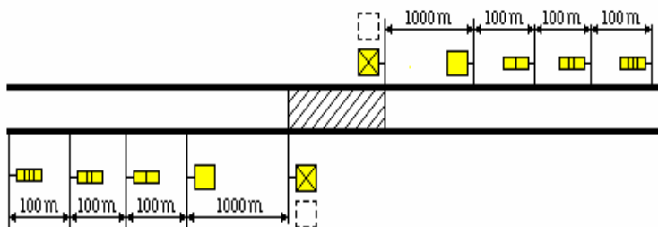
Fig. 115. Schema semnalizării porțiunii de linie slăbită pe linie simplă.
