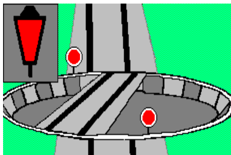
Fig. 175. Intrarea pe placa de întoarcere a locomotivelor sau ieșirea de pe placă este oprită.
