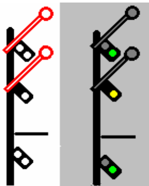
Fig. 18. LIBER pe linie abătută, cu viteza redusă. Semaforul de ieșire sau semaforul de parcurs este pe liber.
