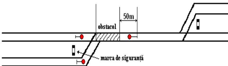
Fig. 3. Acoperirea obstacolului sau a locului de executare a lucrării, dacă acesta se află pe un schimbător de cale.
