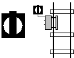
Fig. 170. Trecerea liberă, sabotul de deraiere este răsturnat de pe șină.
