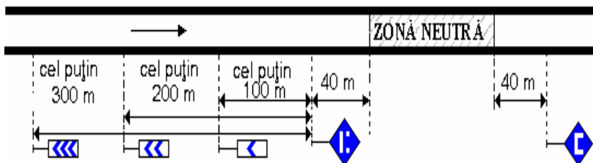
Fig. 199. Amplasarea indicatoarelor și balizelor avertizoare ale zonei neutre a liniei de contact.
