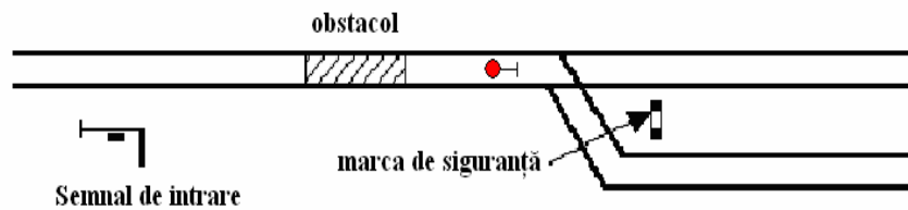
Fig. 6. Acoperirea unui obstacol sau a locului de executare a lucrării, dacă acesta se află între schimbătorul de cale de la intrarea în stație și semnalul de intrare.
