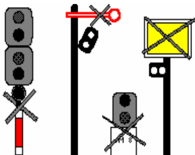
Fig. 53. Exemple de semnale care nu sunt în exploatare.
