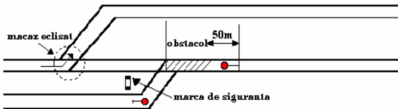
Fig. 4. Acoperirea obstacolului sau a locului de executare a lucrării, dacă acesta se află pe un schimbător de cale, iar în apropierea lui se găsește un alt schimbător de cale, care poate să fie astfel fixat încât să nu permită trecerea materialului rulant spre schimbătorul de cale cu obstacol.
