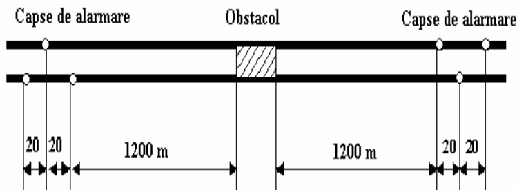
Fig. 1. Schema acoperirii unui obstacol neprevăzut cu capse de alarmare.
