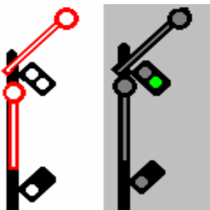
Fig. 7. LIBER în direcția I
