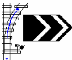
Fig. 167. Macazul este în poziție de abatere la dreapta.
