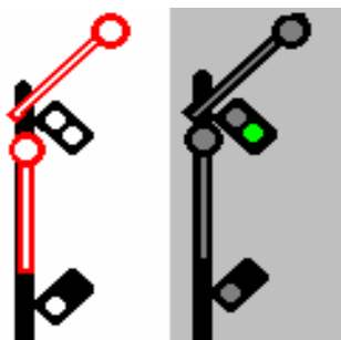
Fig. 2. LIBER pe linia directă.
