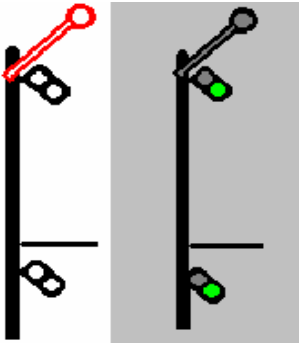
Fig. 21. LIBER cu viteza stabilită. Semaforul de ieșire este pe liber.
