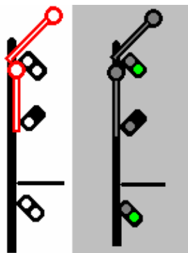
Fig. 16. LIBER pe linia directă, cu viteza stabilă. Semaforul de ieșire sau semaforul de parcurs este pe liber.
