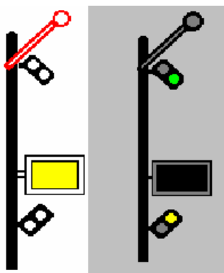
Fig. 20. LIBER cu viteza stabilită. ATENȚIE! Semaforul de ieșire ordonă oprirea.
