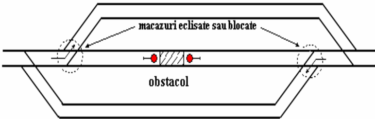
Fig. 1. Acoperirea obstacolului sau a locului de executare a lucrării, care se află pe o linie din incinta stației.
