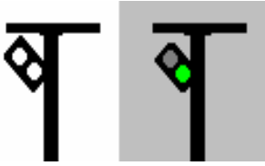
Fig. 10. LIBER cu viteza stabilită. Semaforul următor este pe liber pe linia directă.
