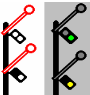
Fig. 8. LIBER în direcția II
