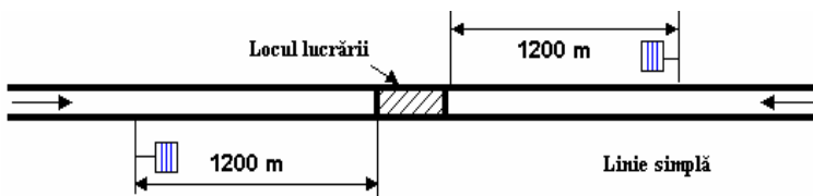
Fig. 122. Schema semnalizării locurilor de executare a lucrărilor pe linie curentă simplă.
