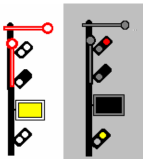
Fig. 14. OPREȘTE fără a depăși semnalul!
