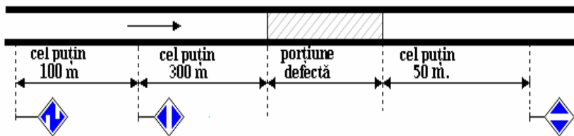
Fig.203. Amplasarea indicatoarelor de acoperire a porțiunii liniei de contact pe care este interzisă circulația locomotivelor electrice cu pantograful ridicat.
