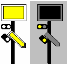
Fig.12. LIBER cu viteza stabilită. Semaforul următor este pe liber pe linie abătută, cu viteza redusă.
